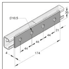
Łącznik 35/4 z 4 otworami
