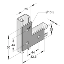
Łącznik płaski 35/4 typ L
