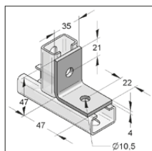
Łącznik kątowy 35/4 z 2 otworami
