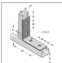
Łącznik kątowy 35/4 z 4 otworami 90°
