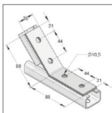
Łącznik kątowy 35/4 z 4 otworami 135°
