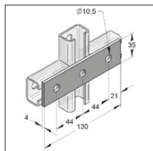
Łącznik 35/4 z 3 otworami
