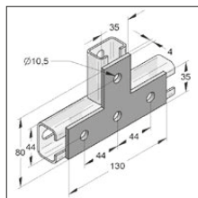
Łącznik płaski 35/4 typ T
