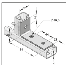
Łącznik kątowy 35/4 z 3 otworami
